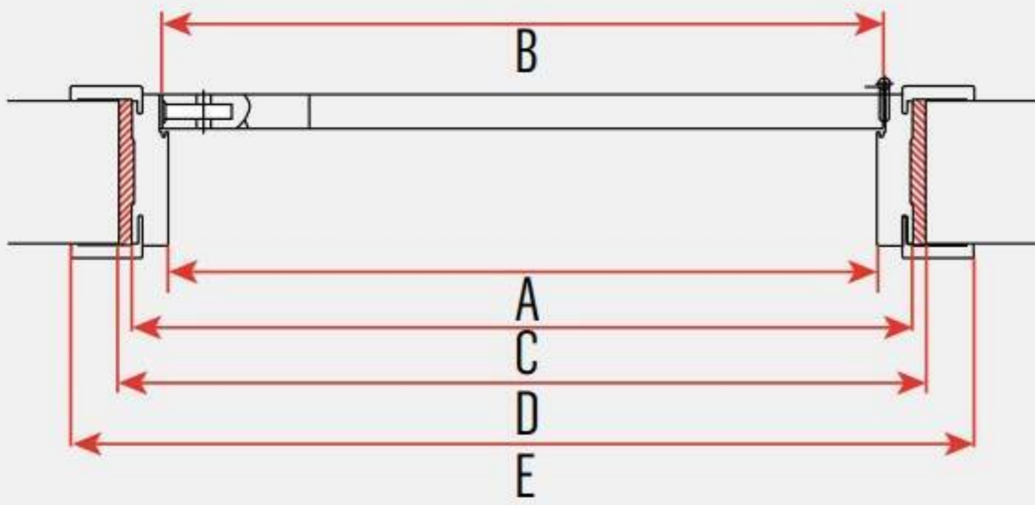
RESİM 1: KAPI GENEL KESİT
