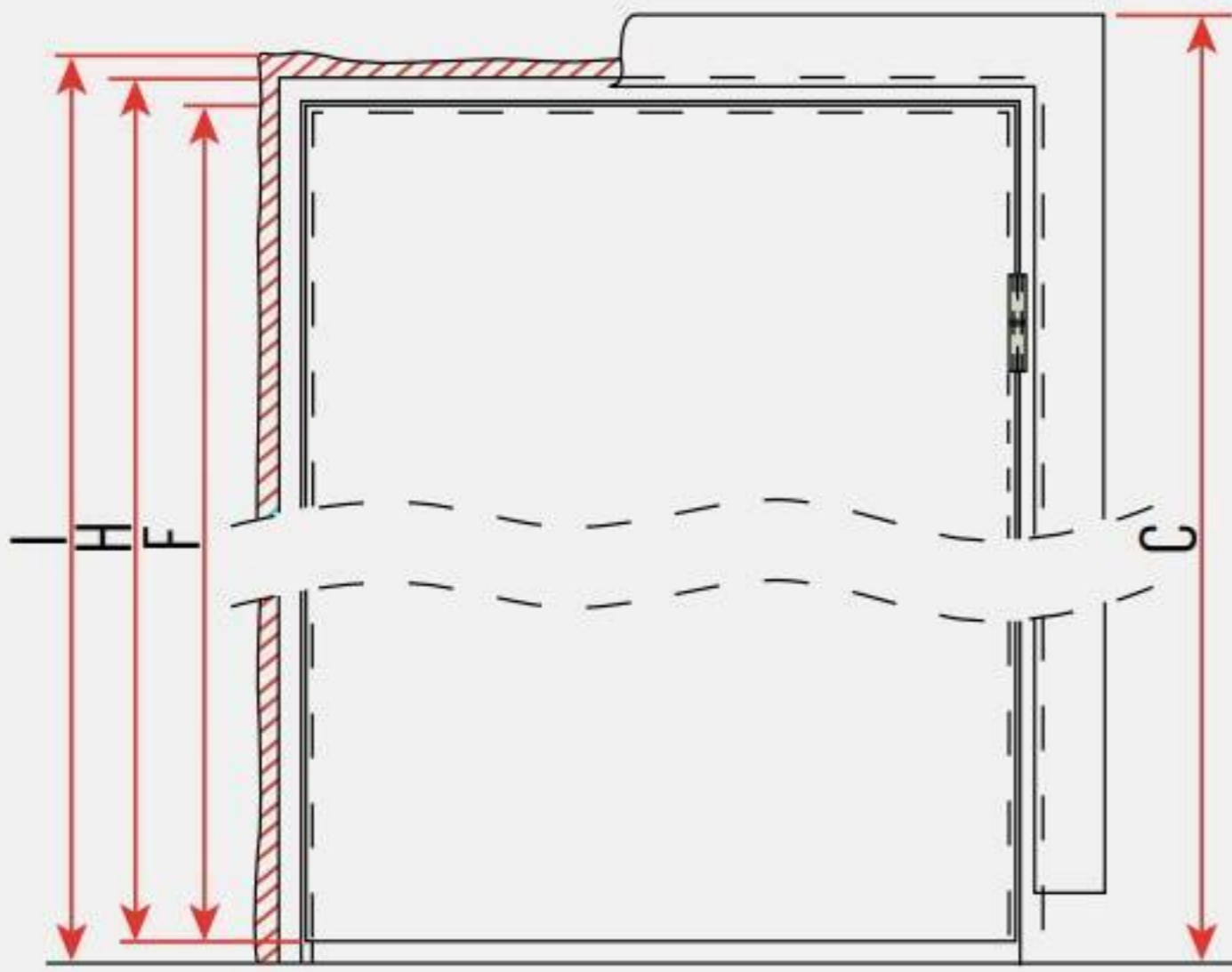
RESİM 2: KAPI YÜKSEKLİKLERİ
