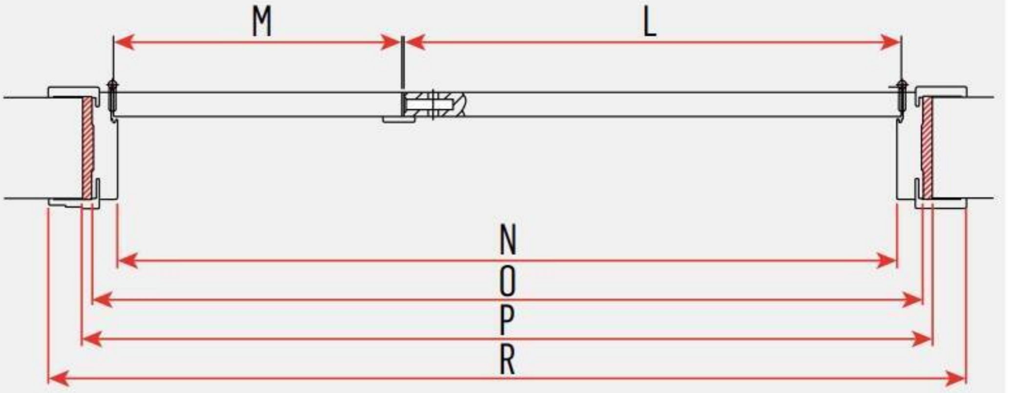
RESİM 3: SALON KAPISI GENEL KESİT
